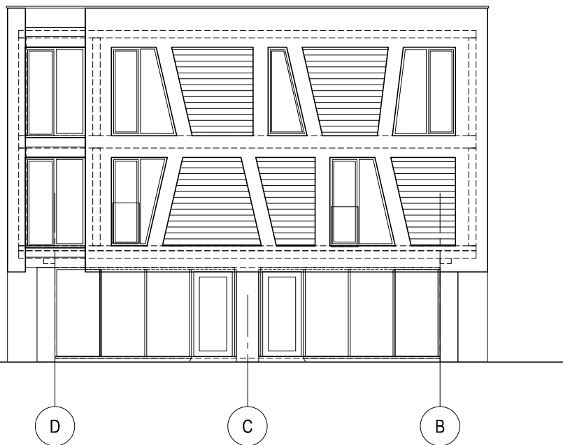
Šiaurės fasadas
